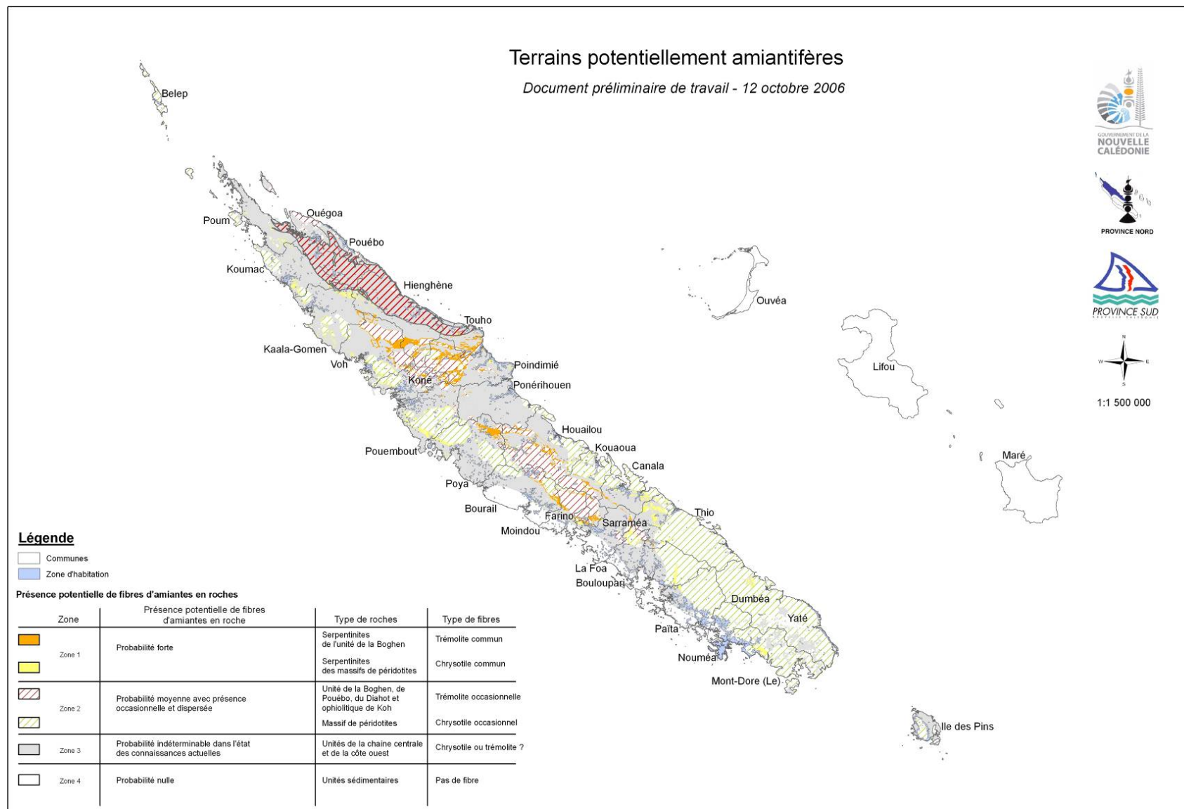
Figure 2 - Cartographie des terrains potentiellement amiantifères en Nouvelle-Calédonie.
